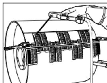
Přiložíme pásek a zavaříme
